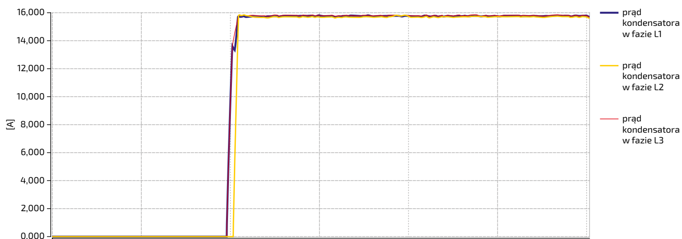
Przebieg RMS 10 ms załączenia rozładowanego kondensatora poprzez tłącznik LH
