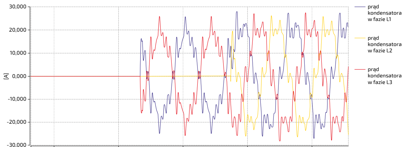
Przebieg oscyloskopowy załączenia rozładowanego kondensatora poprzez tłącznik LH w mocno zniekształconej sieci
