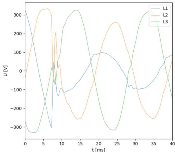
Napięcia sieci
